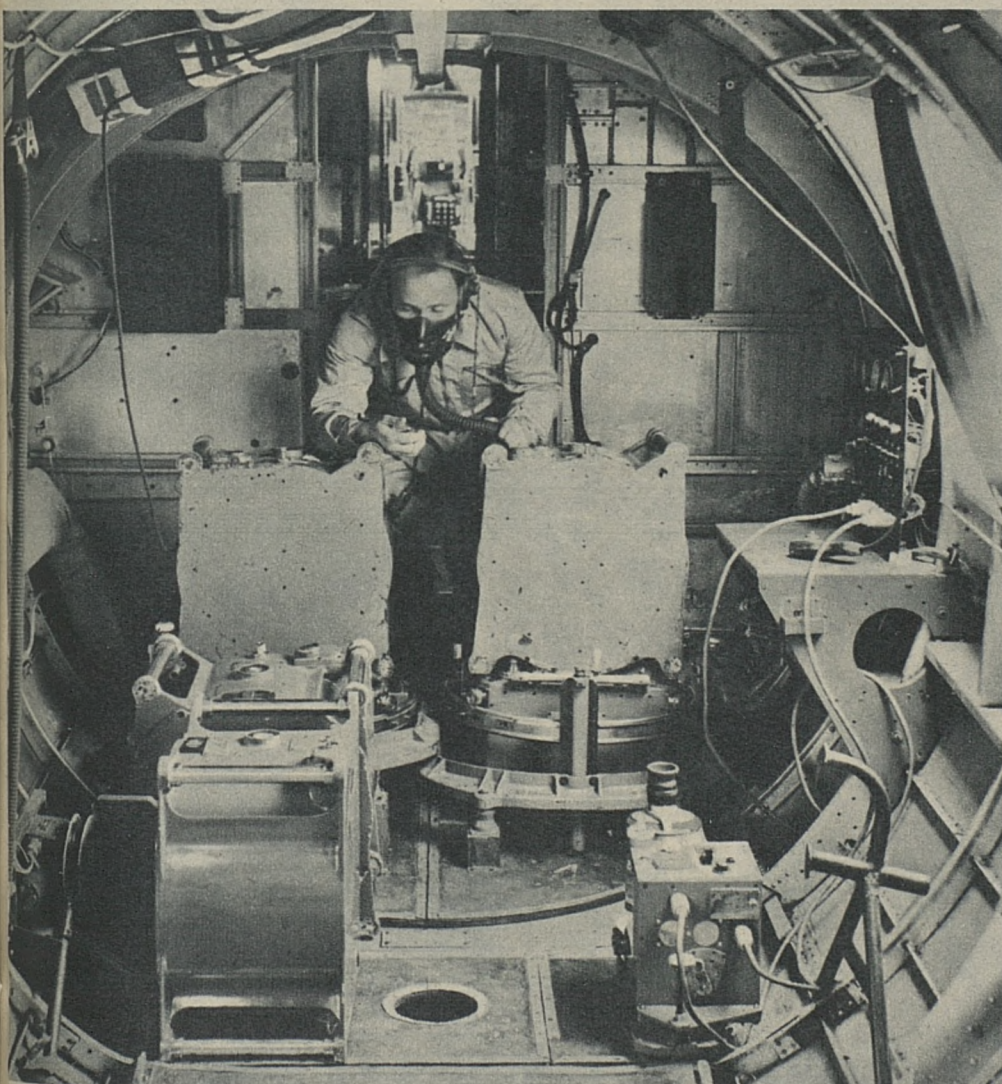
A bord d'une forteresse volante, l'opérateur ne se trouve pas dans le nez de l'appareil, mais dans la carlingue. Il s'apprête à mettre ses appareils en marche sur l'ordre du navigateur.
