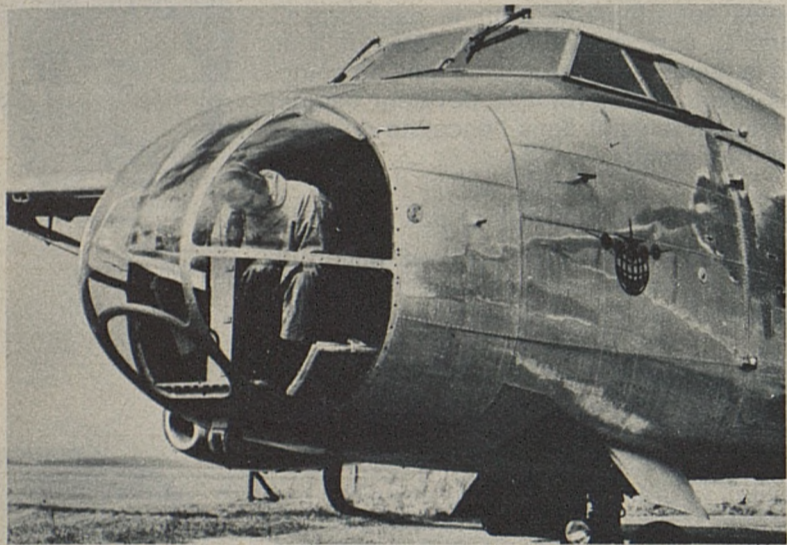
Dans le nez vitré d'un Hurel-Dubois H-34 (l'IGN est le seul à utiliser cet avion, puisqu'il en a acheté une série de huit appareils), le navigateur est penché sur son viseur prismatique.
